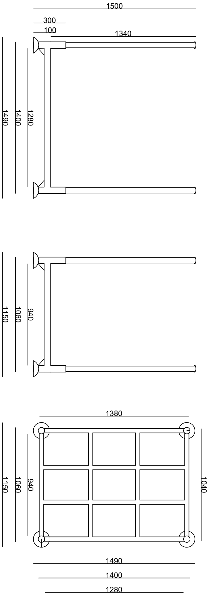
MP093-03 PEDANE / PALLET CON MONTANTI LIBERI REMOVIBILI (NUOVI)
