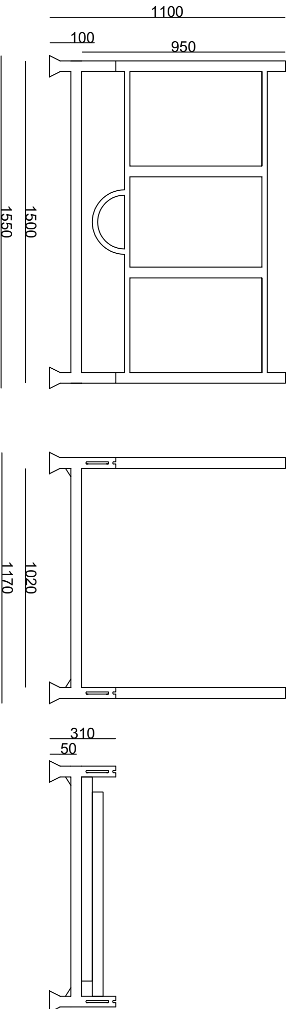
MP093-01 PALLET PORTA ROTOLI ripiegabile mm1550x1170 h1100 kg.60 +/-5% (nuovi)
