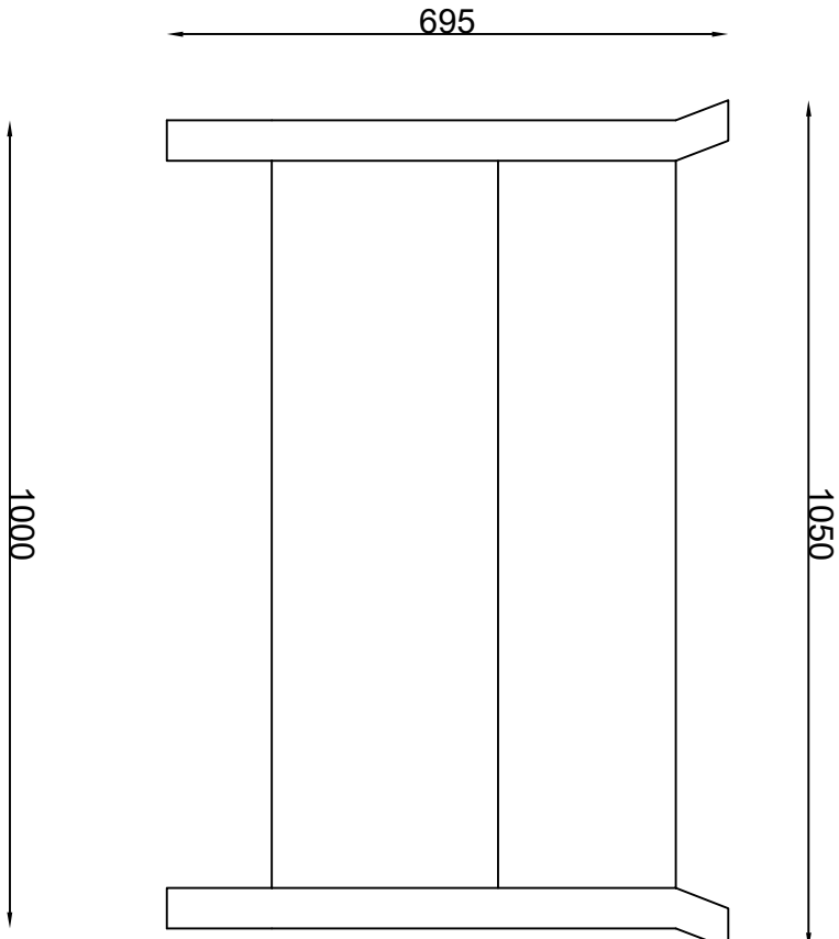
MC036-22: Contenitore in lamiera a BOCCA di LUPO portata 1000 kg
